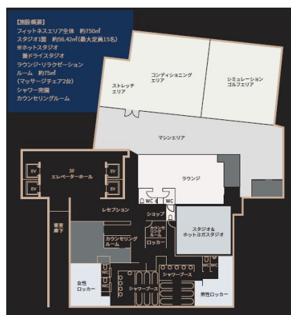
フィットネスルキナ熱海平面図
